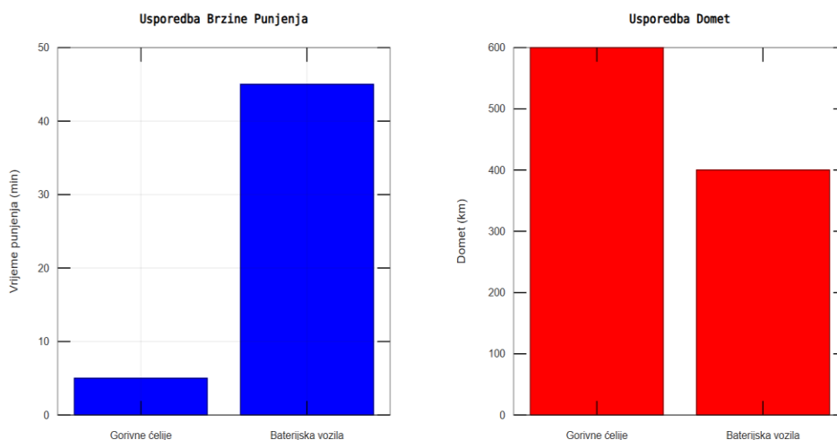
Slika 4. Usporedba brzine punjenja i dometa između vozila s gorivim ćelijama i baterijskih električnih vozila.
