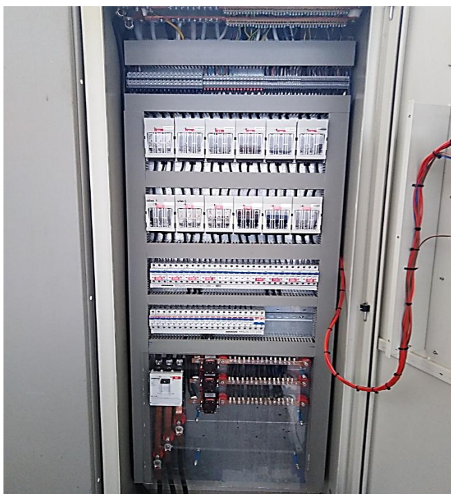
Slika 4. Gotov razvodni ormar
