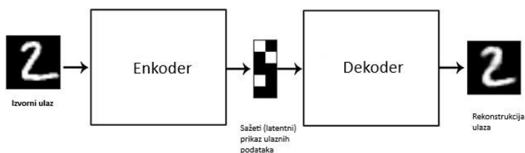
Slika 1. Primjer općenite arhitekture neuronske mreže autoenkodera
