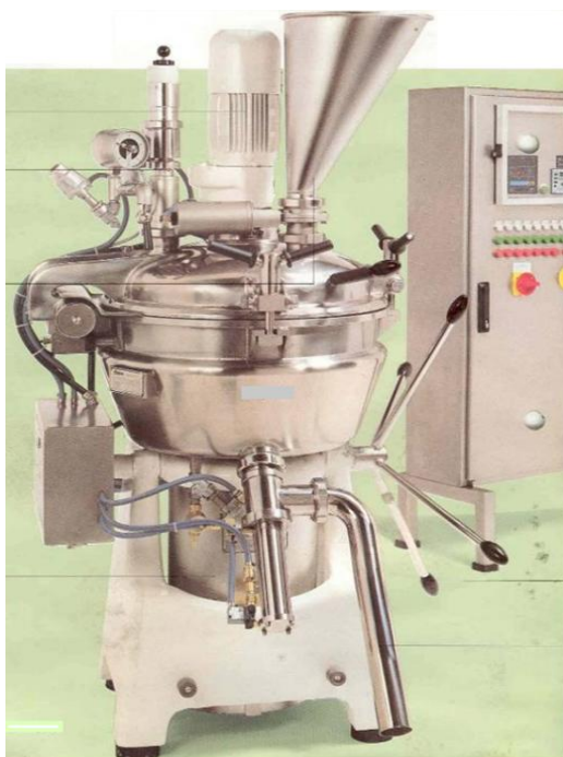
Slika 1. Stroj u proizvodnji hrane [1]
