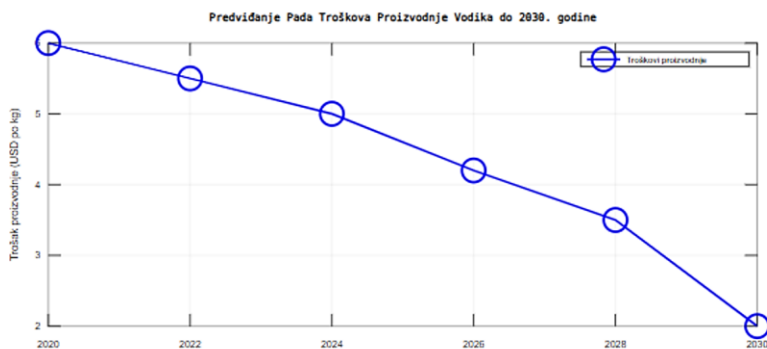
Slika 6. Predviđanje pada troškova proizvodnje vodika do 2030. godine
