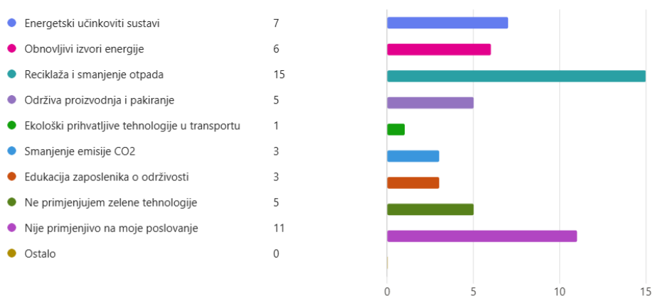
Slika 5. Implementirane zelene tehnologije
