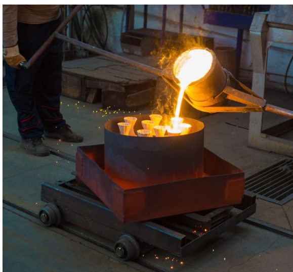
Slika 1. Ručno izlivanje rastopljenog metala u kalupe
