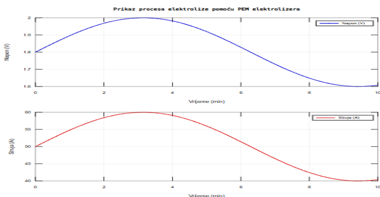
Slika 3: Simulacija procesa elektrolize pomoću PEM elektrolizera s napajanjem iz obnovljivih izvora energije putem platforme https://octave-online.net/ .
