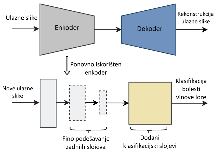
Slika 2. Prikaz postupka primjene autoenkodera
