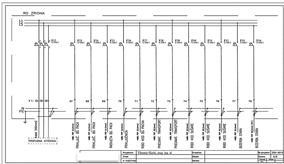
Slika 3. Tropolna shema ormara – peta stranica scheme
