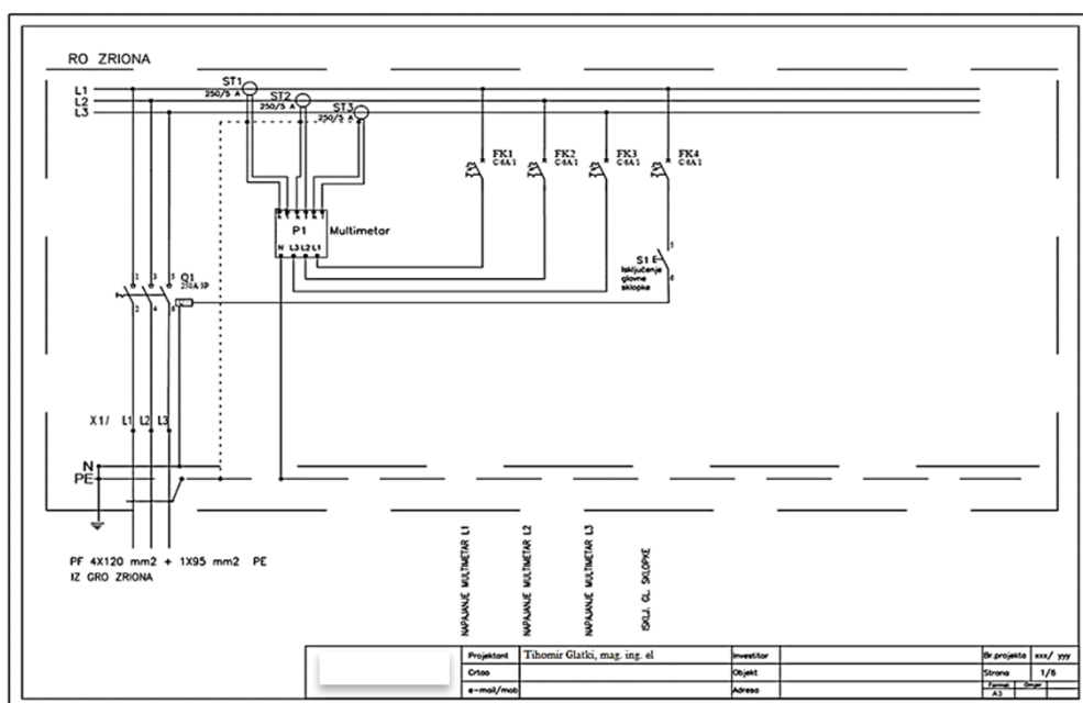
Slika 2. Trolpolna shema ormara – prva stranica sheme
