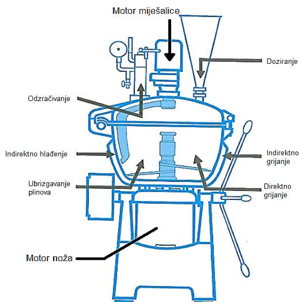
Slika 2. Osnovni dijelovi stroja u proizvodnji hrane [1]
